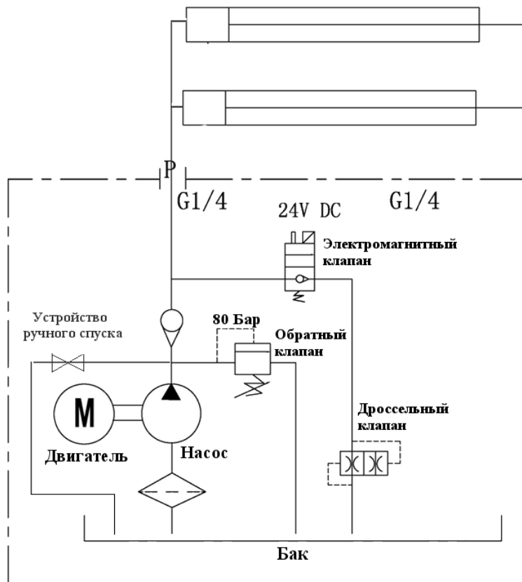
Рисунок 3. Схема гидравлическая
