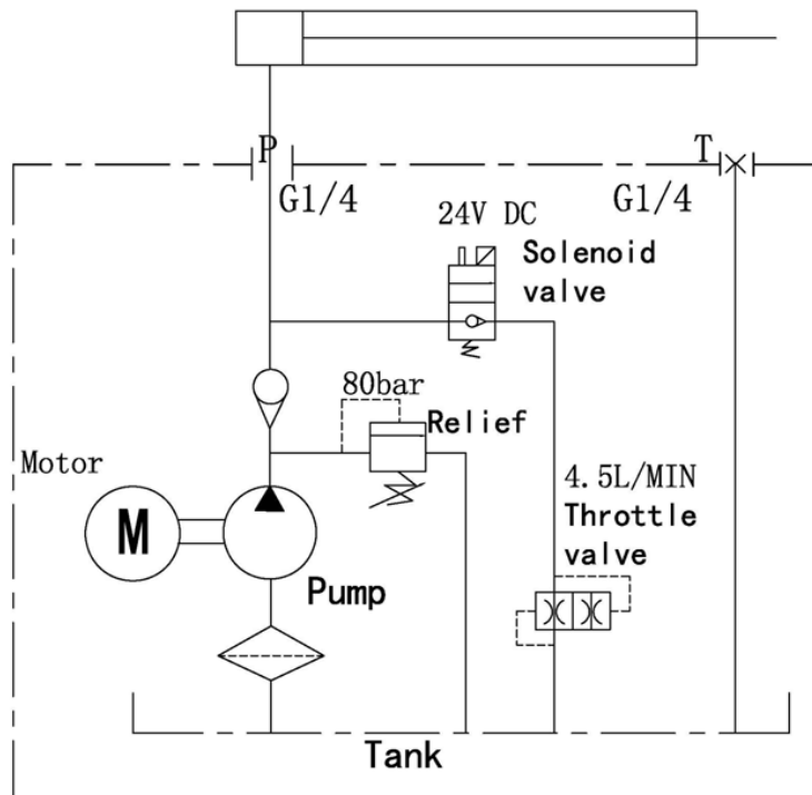
Рисунок 3. Схема гидравлическая
